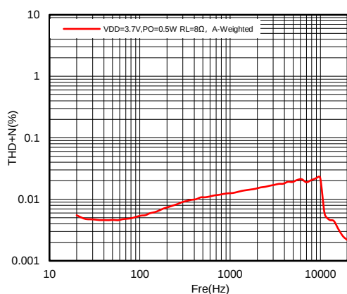
图7 频率失真曲线
