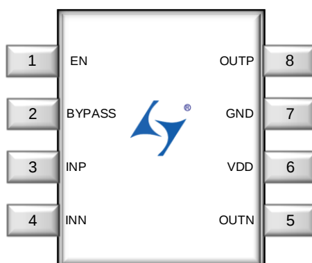
图2. LTK5150管脚图
