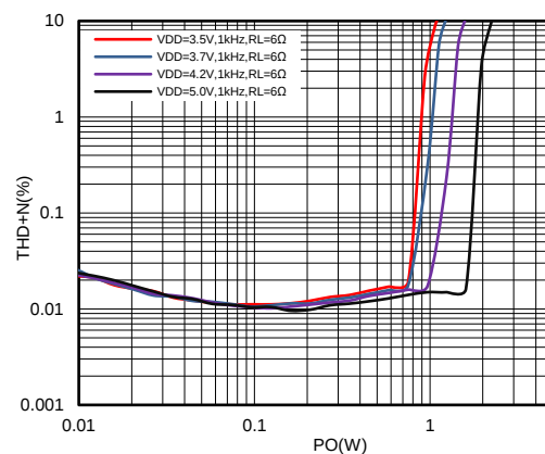
图4 6Ω负载下不同电源电压的的功率曲线
